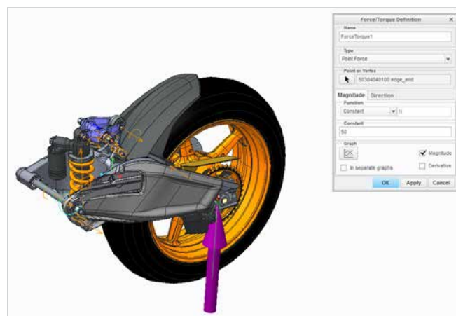
Приложение динамических усилий к сборке с помощью PTC Creo MDO для оптимизации качества.
